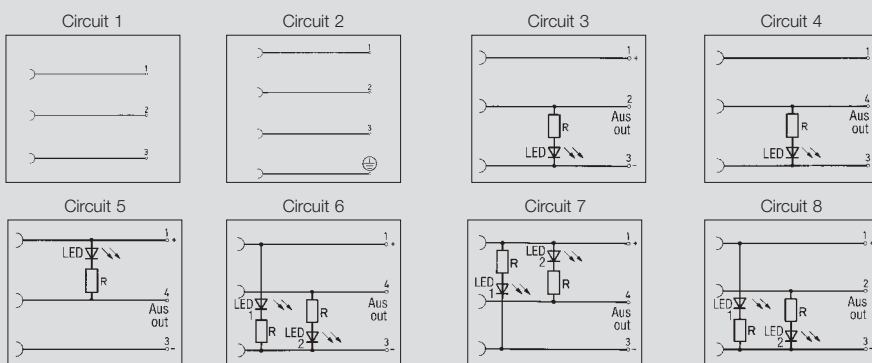
Wiring scheme
