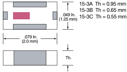
Case 15-3 (EIA 0805 / 2012)
