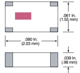
Case 15-4 (EIA 0805 / 2012)
