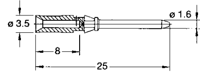
Stiftkontakt/Pin contact
