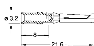
Buchsenkontakt/Socket contact
